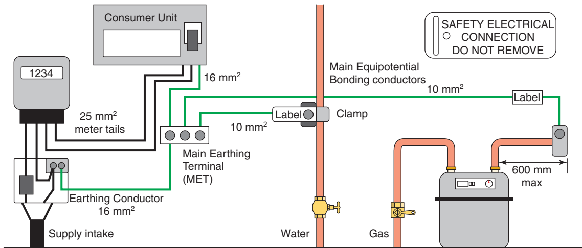
Figure 9.15 Equipotential bonding
